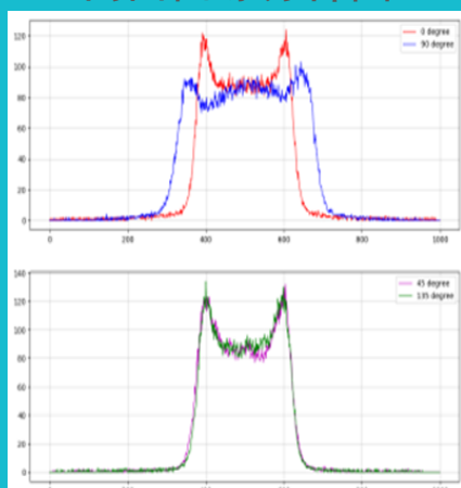
剖面曲線分佈圖
